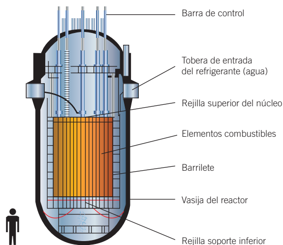
Esquema de un reactor nuclear PWR
