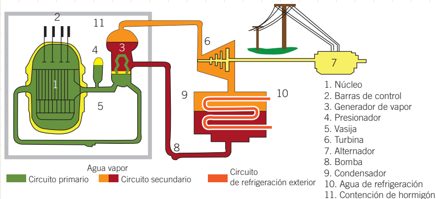
Esquema de una central de agua a presión
