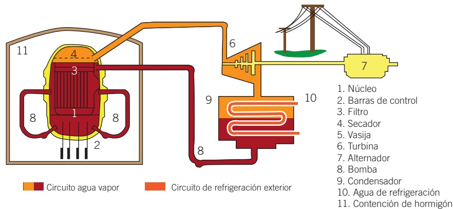
Esquema de funcionamiento de una central nuclear (BWR)
