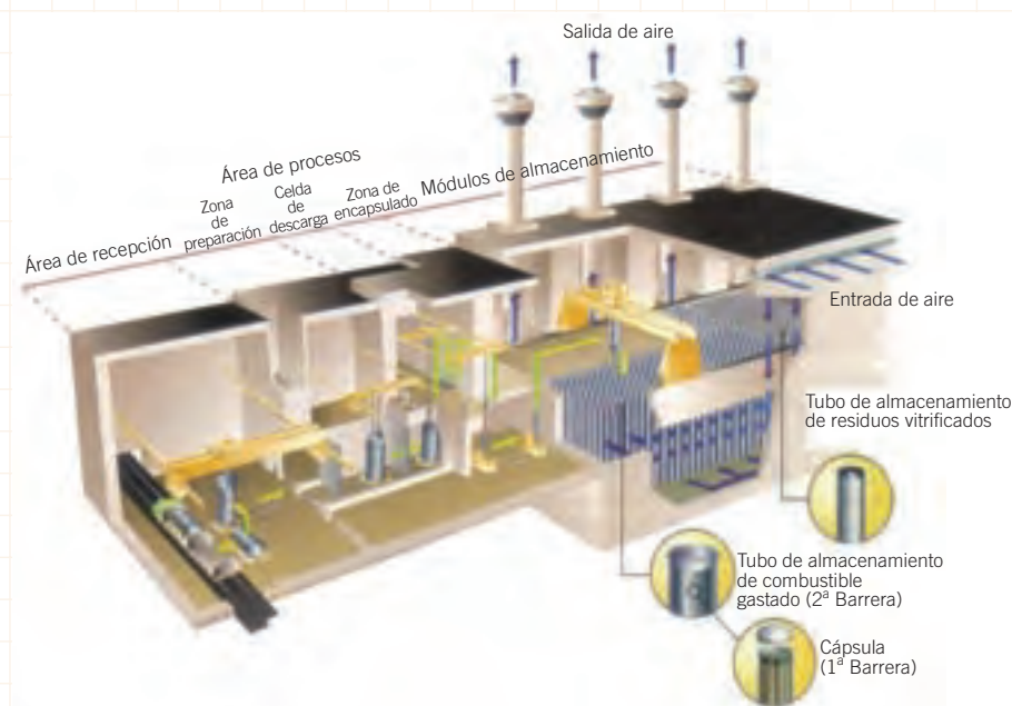
Esquema de ATC. Cámaras
